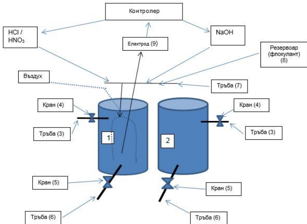
Фиг.1 – Принцилна схема физико-химично третиране чрез коагулацията на водни разтвори, емулсии и суспензии посредством коагуланти и флокуланти, променящи тяхното рН
